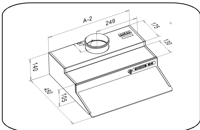
Fläktdel för köksfläkt DTT-200
