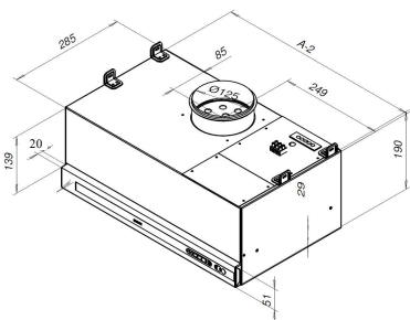
ilmanvaihtokoneet Talteri DIVK
