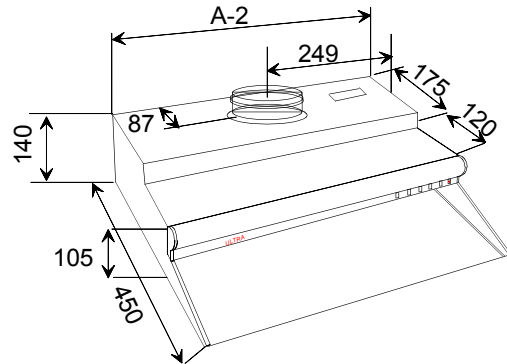
Liesikuvun puhallinosa DTT-200
