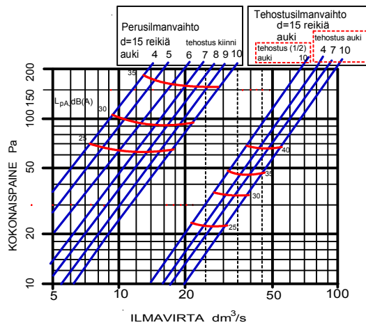
ilmavaihtokoneet Talteri DIVK
