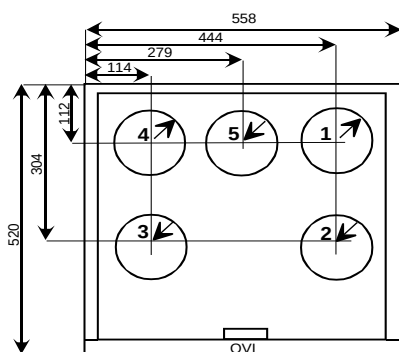
korkeus 495 mm
