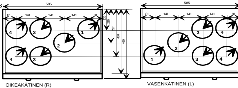
Asennus sarja 1
